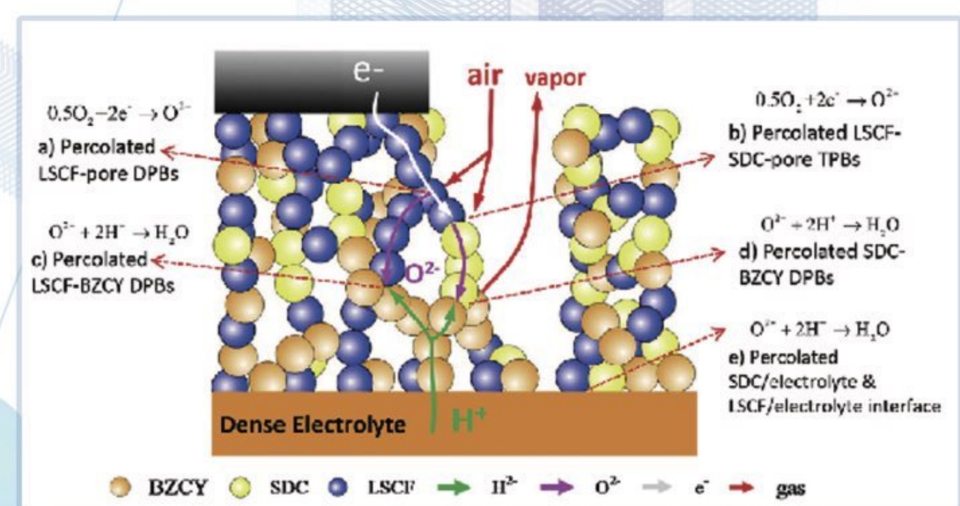
LSCF-SDC-BZCY 理论模型 (J. Power Sources 2016, IF: 8.247)
